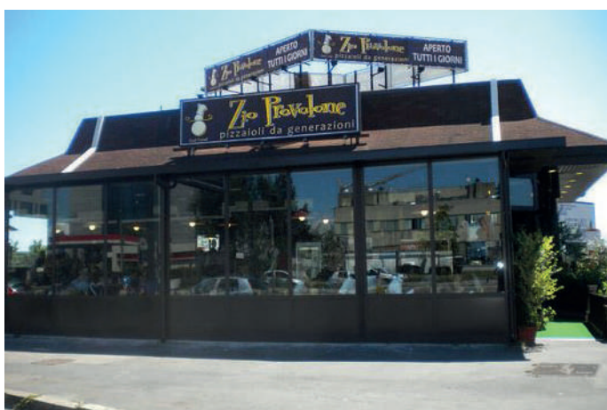
Milano (zona Lorenteggio) Ristorante Zio Provolone Rooftop da 26 kW
